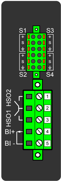
Figure. 7.5.4 - 195. Arc protection module.
