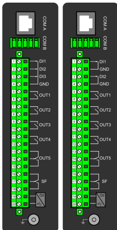
Figure. 7.2 - 187. CPU module.
